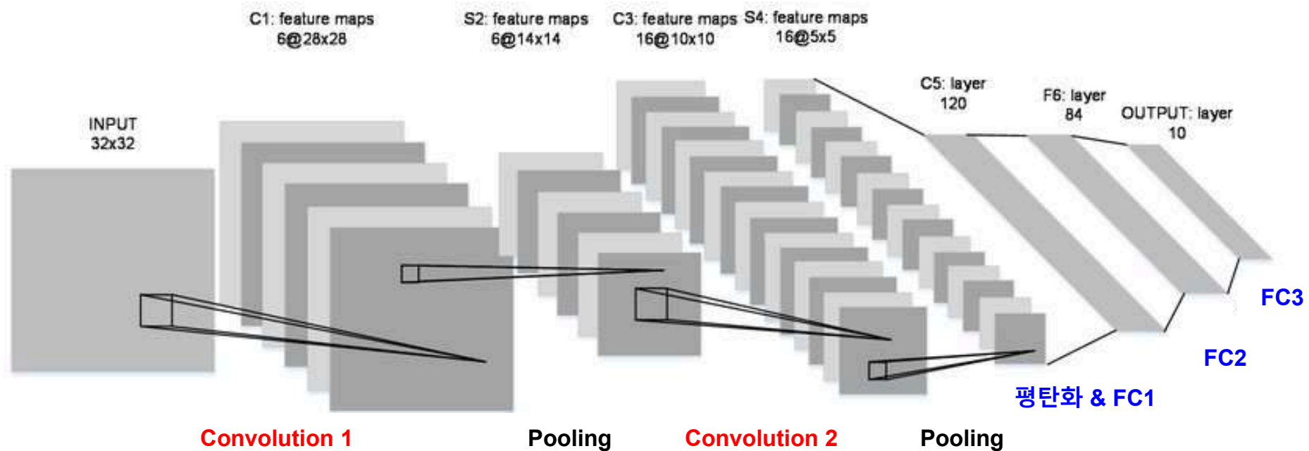
LeNet-5 구조
